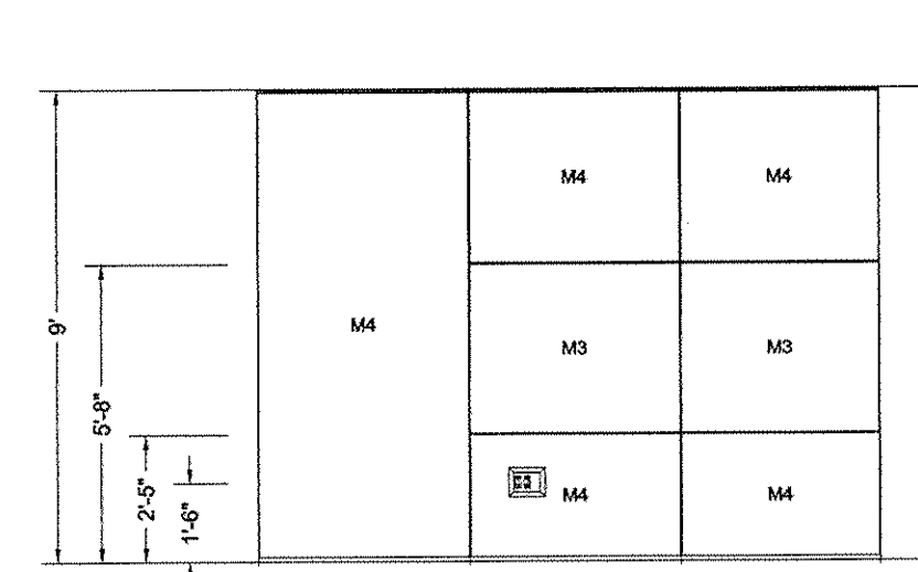
Elevation N
