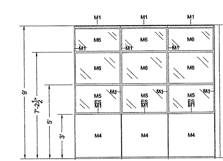
Elevation Z
