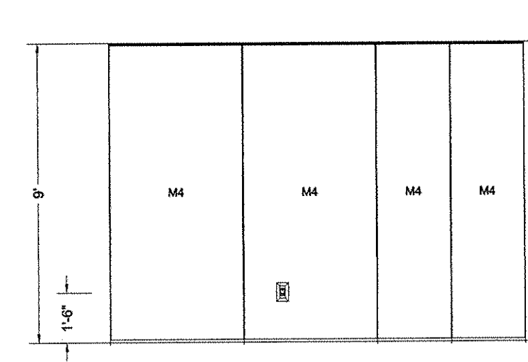
Elevation J
