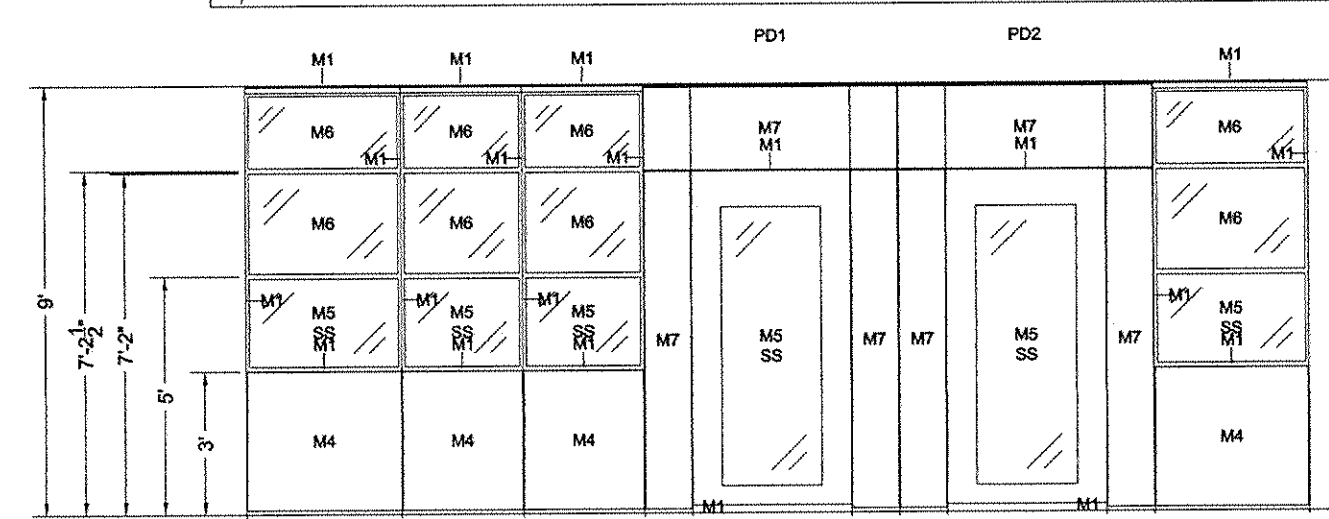
Elevation G
