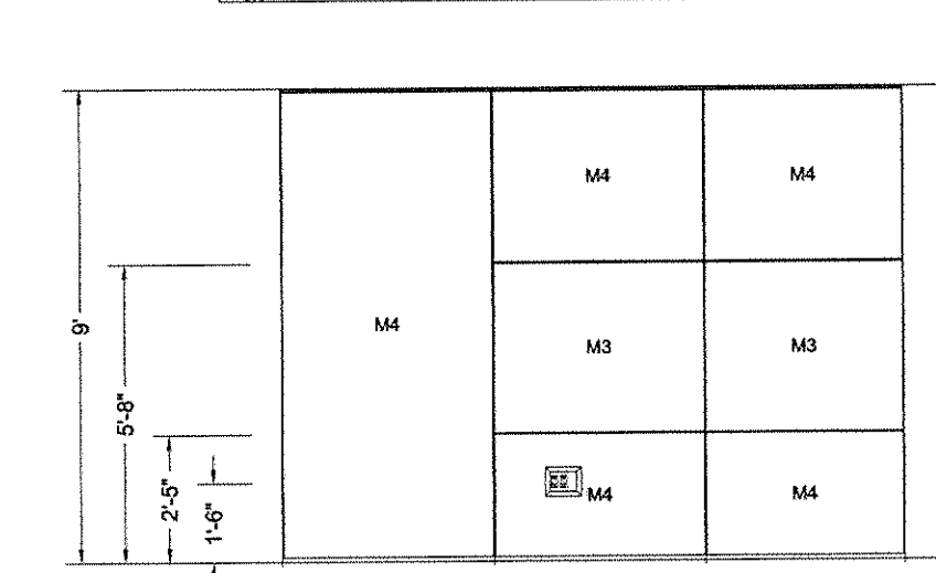
Elevation U
