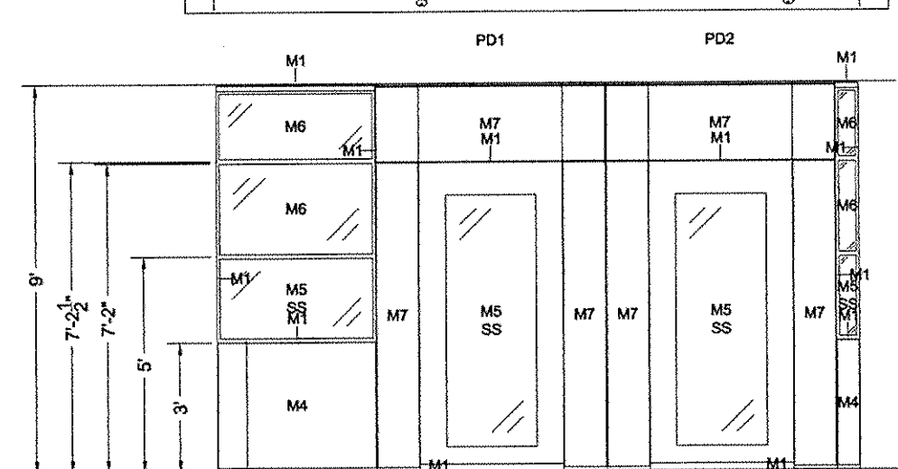
Elevation A
