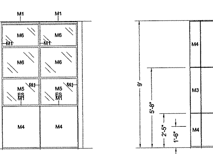
Elevation AB
