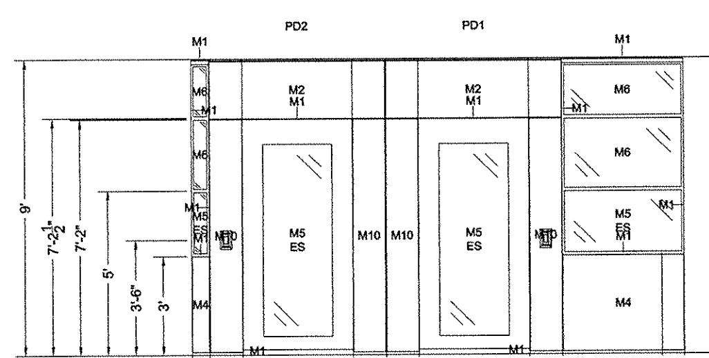
Elevation B
