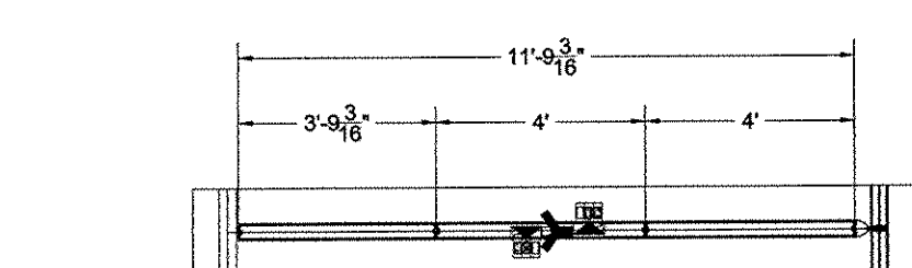
Elevation G
