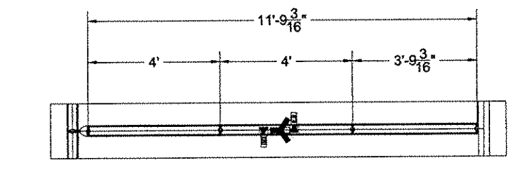
Elevation J
