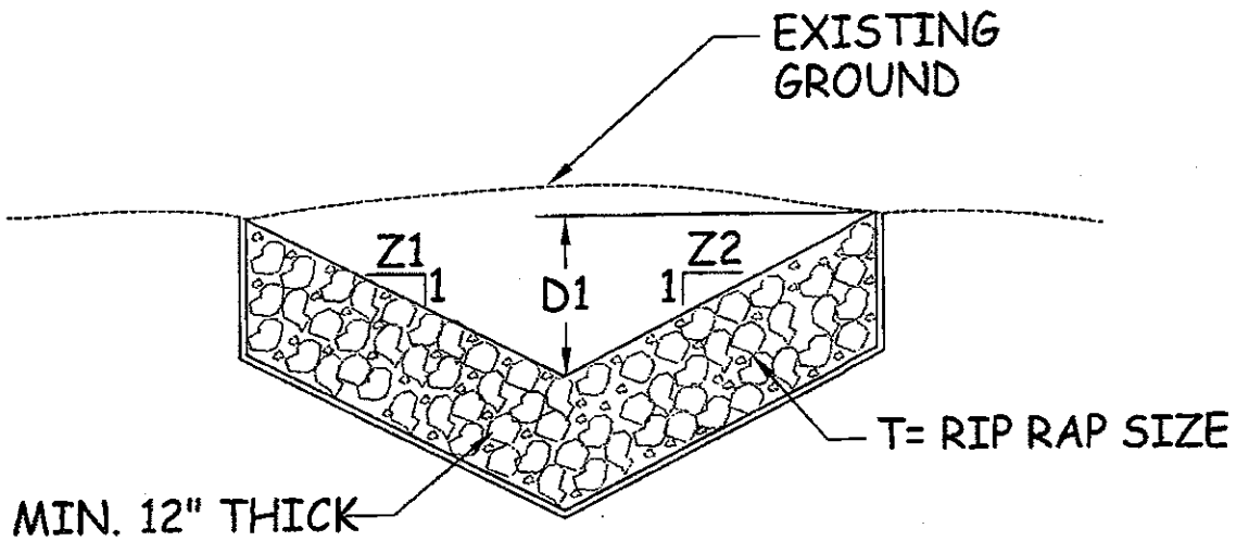
TYPICAL SECTION DIVERSION DITCH N.T.S.
