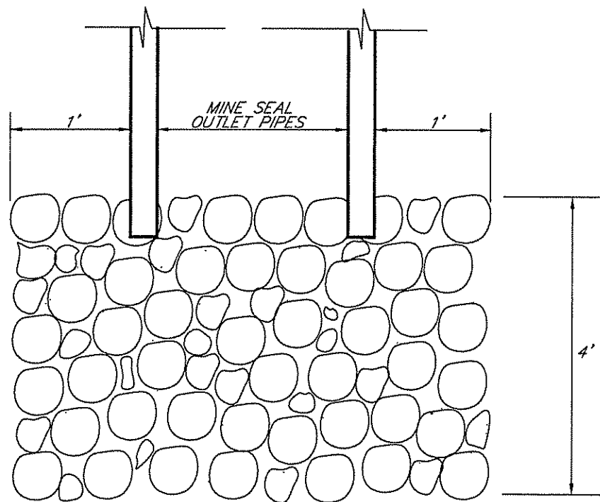
ROCK RIPRAP SPLASH PAD
