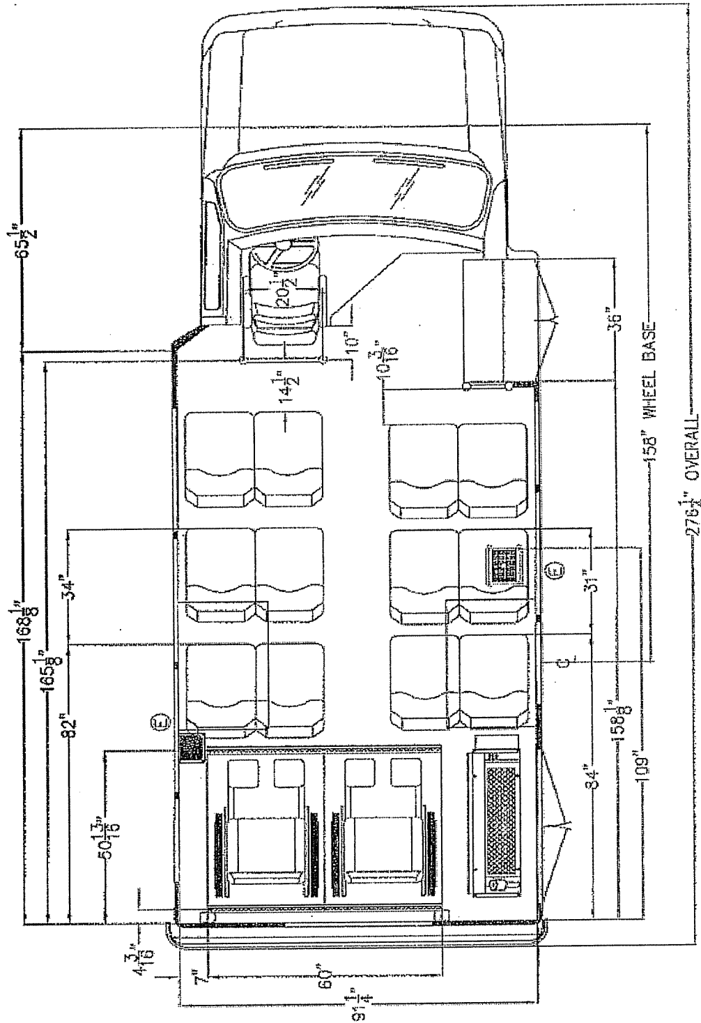
12 Passenger, 2 W/C Spaces
