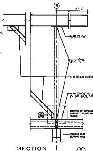
SECTION SCALE: 3/4" = 1'-0"
