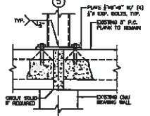
DETAIL SCALE: 1-1/2" = 1'-0"
