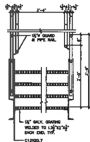
SECTION SCALE: 3/4" = 1'-0"
