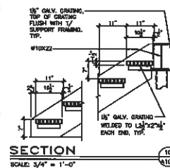
SECTION SCALE: 3/4" = 1'-0"
