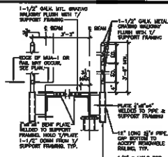
SECTION SCALE: 3/4" = 1'-0"
