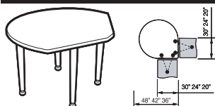
Teardrop 90° Table
