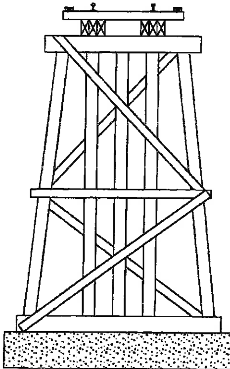
BENT 8-16
