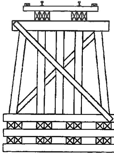
BENT 2-7, 18, 19
