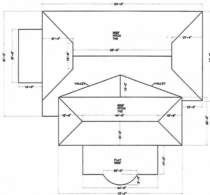
MEDICAL BUILDING ROOF DETAILS N. T. S.
