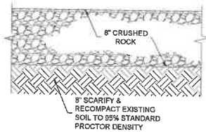
A1 TYPICAL GRAVEL SECTION N.T.S.
