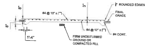
SECTION A-A N.T.S.
