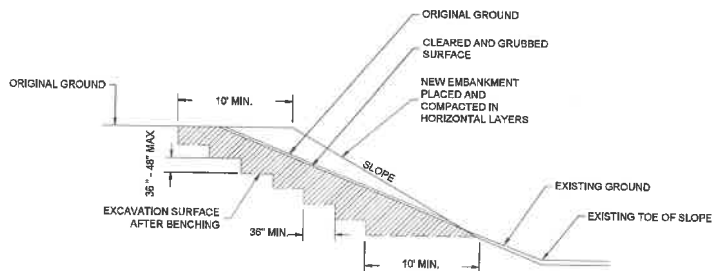
A3 SLOPE STABILITY DETAIL N.T.S.
